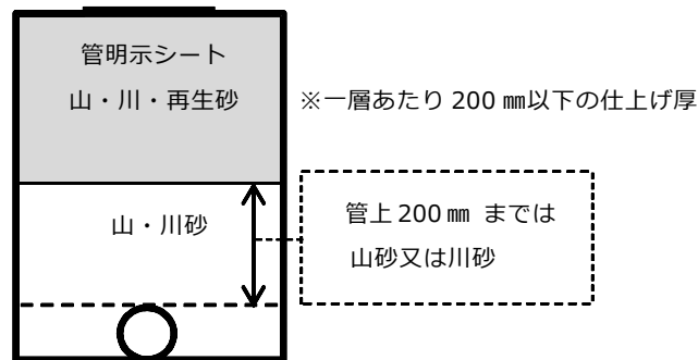
図 8-1…埋戻し工事概略図
