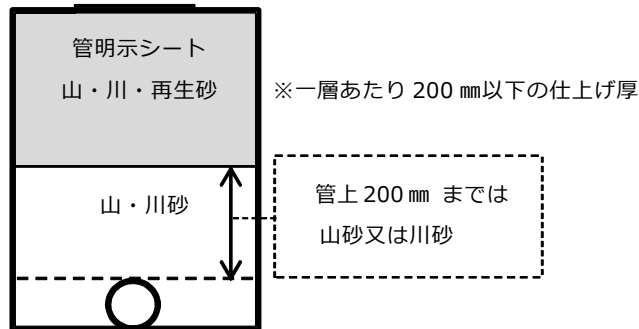
図 9-1…埋戻し工事概略図
